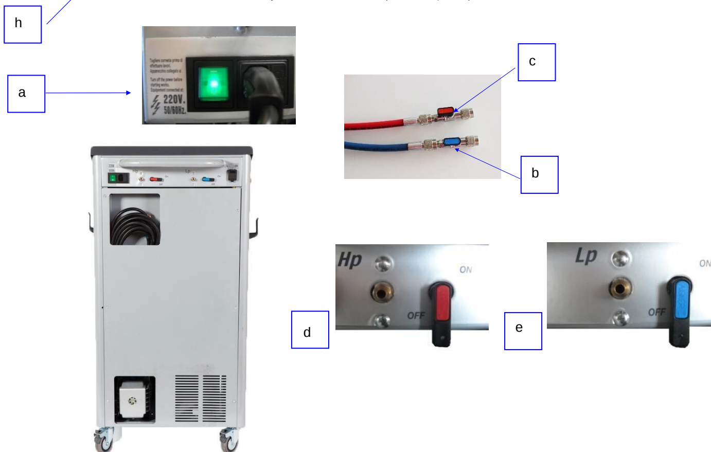
Рисунок 6 – Станция (вид спереди)
